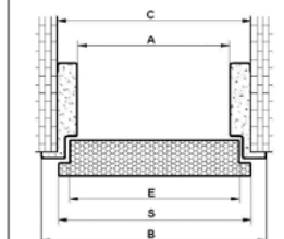
Rysunek poglądowy dla ościeżnic FN, FT PREMIUM, FT SL, FT SL PREMIUM
