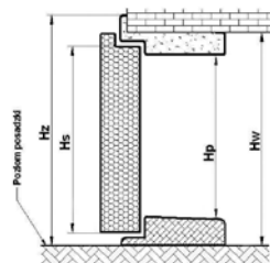
Rysunek poglądowy dla ościeżnic drzwi i progów dla: FN, FT SL, FT PREMIUM, FT SL PREMIUM
