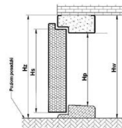
Rysunek poglądowy dla ościeżnic drzwi i progów dla: FD, FC, FR, FR SL, FA SL, FA SL PREMIUM, FR SL PREMIUM, FR PREMIUM, FC PREMIUM
