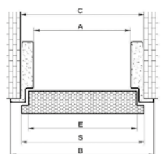
Rysunek poglądowy dla ościeżnicy: FTP SL
