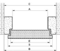
Rysunek poglądowy dla ościeżnic: FAP SL, FRP SL, ALUTERM, FA SL z przekładką
